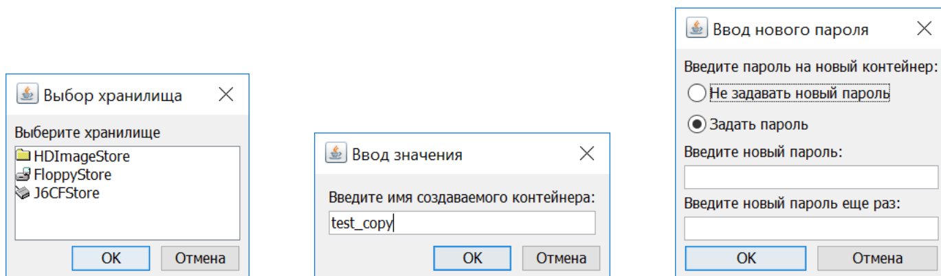
Рисунок 38. Копирование контейнера
